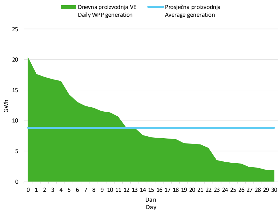
Slika 6 Krivulja trajanja dnevne proizvodnje vjetroelektrana u svibnju 2026. godine
