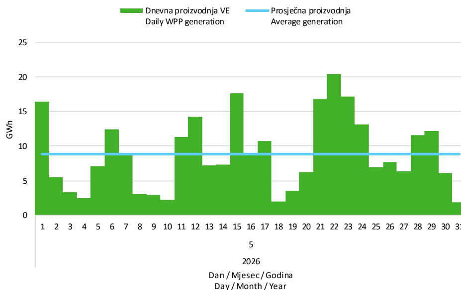
Slika 5 Dnevna proizvodnja svih vjetroelektrana u svibnju 2026. godine
