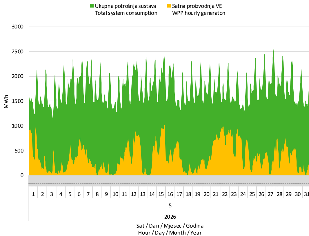
Slika 7 Usporedba satnog dijagrama opterećenja sustava i proizvodnje vjetroelektrana u svibnju 2026. godine
