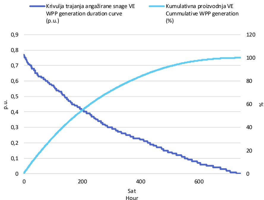
Slika 3 Krivulja trajanja angažirane snage svih VE i kumulativna proizvodnja VE u svibnju 2026. godine u jediničnim vrijednostima
