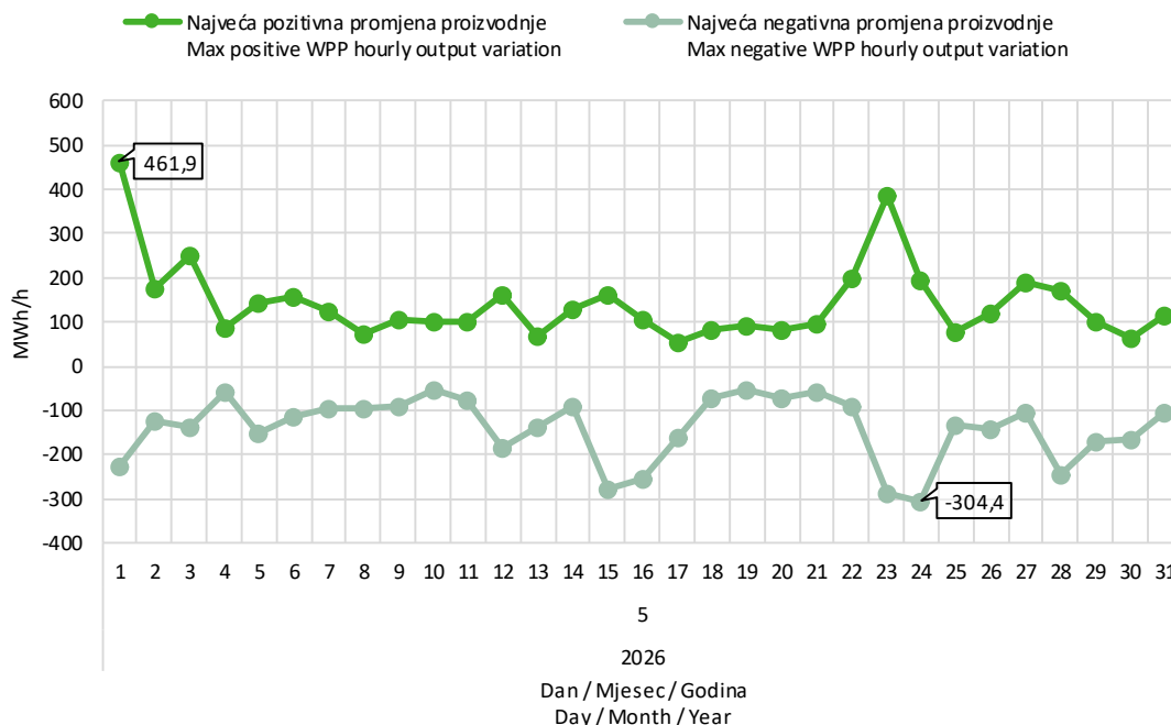
Slika 9 Maksimalna pozitivna i maksimalna negativna promjena satne proizvodnje VE u svibnju 2026. godine
