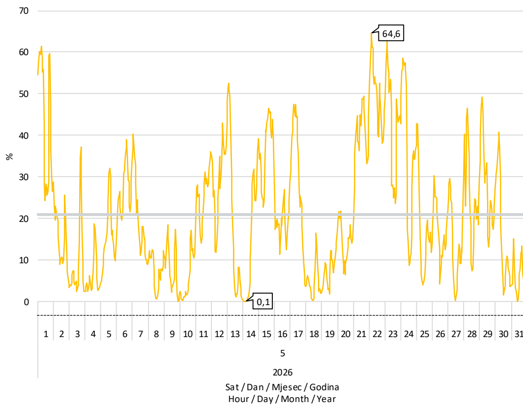
Slika 8 Udio proizvodnje vjetroelektrana u pokrivanju satnog opterećenja elektroenergetskog sustava u svibnju 2026. godine
