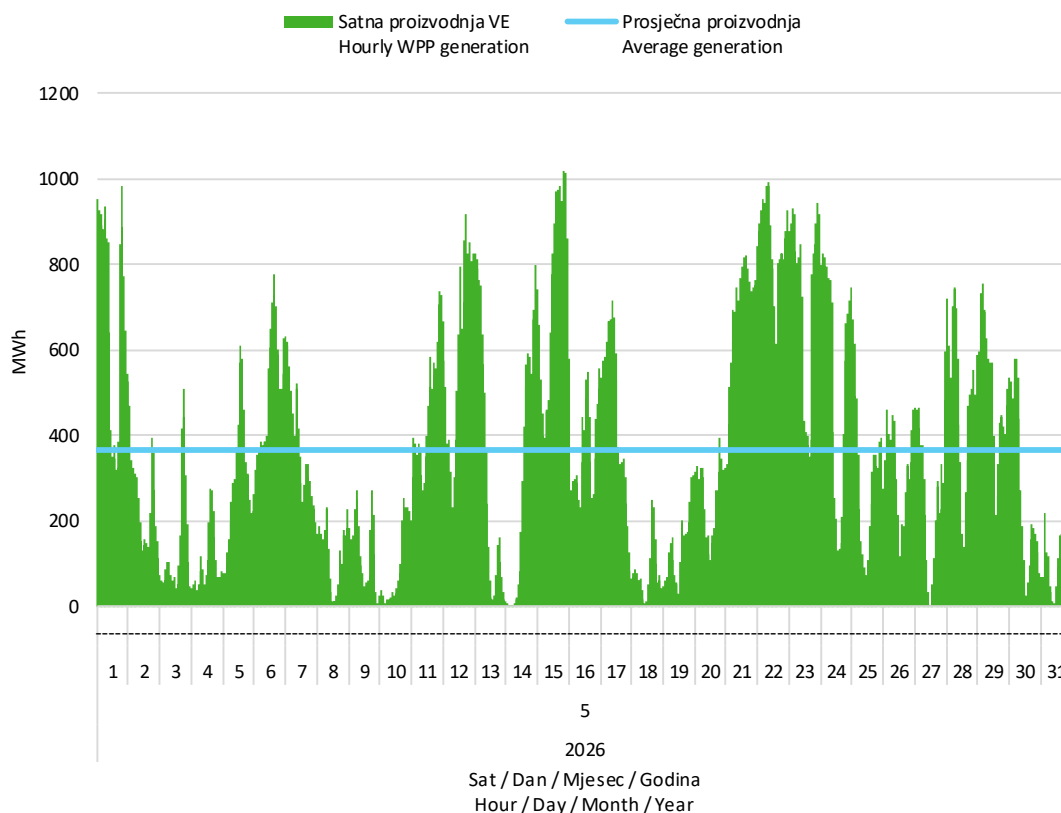
Slika 2 Satna proizvodnja svih vjetroelektrana u svibnju 2026. godine
